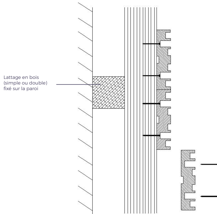
Fig. 1 : Coupe horizontale
